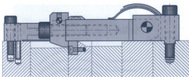
合模状态
