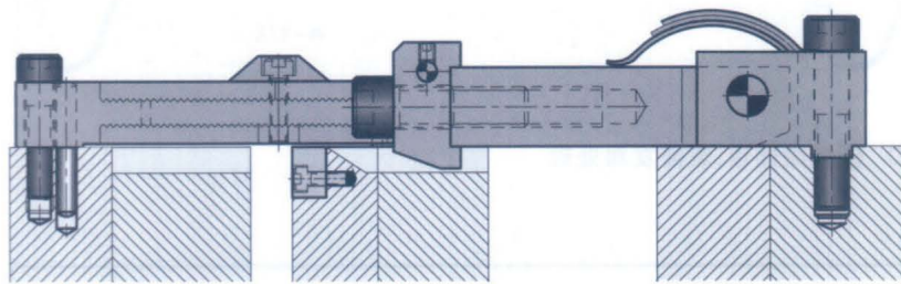
第二次开模
